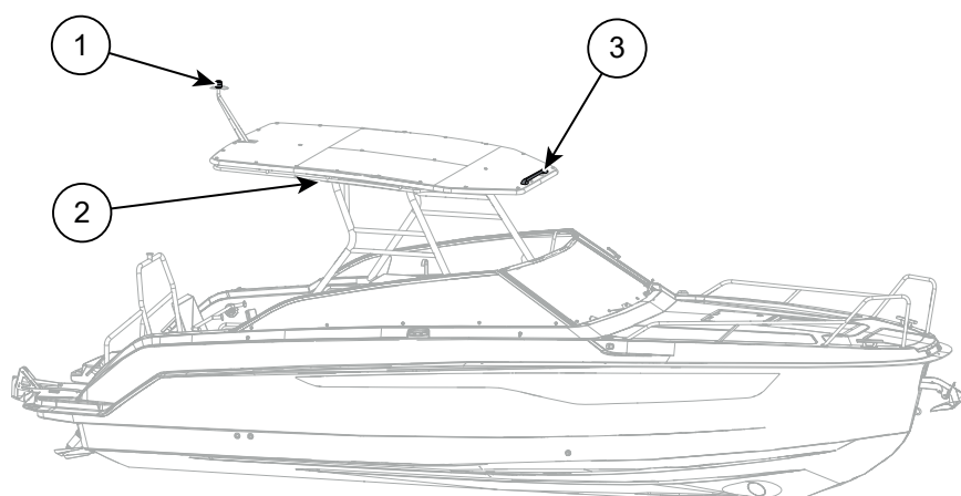
Figur 8.4 Elektrisk utrustning för T-top (tillval)
