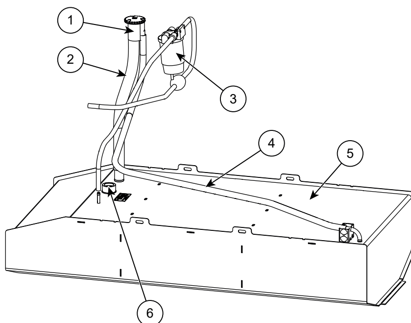
Figur 6.1 Bränslesystem
