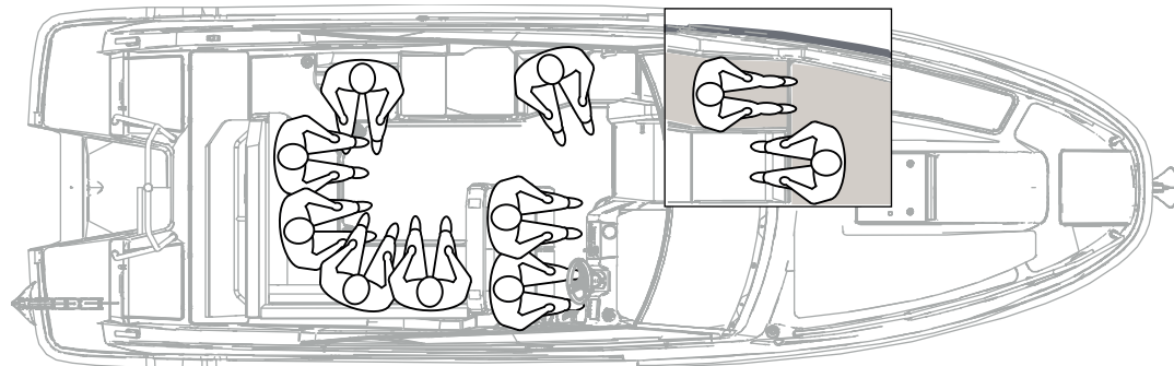
Figur 4.1 Yamarin 80 DC sittplatser för maximalt tio (10) passagerare
