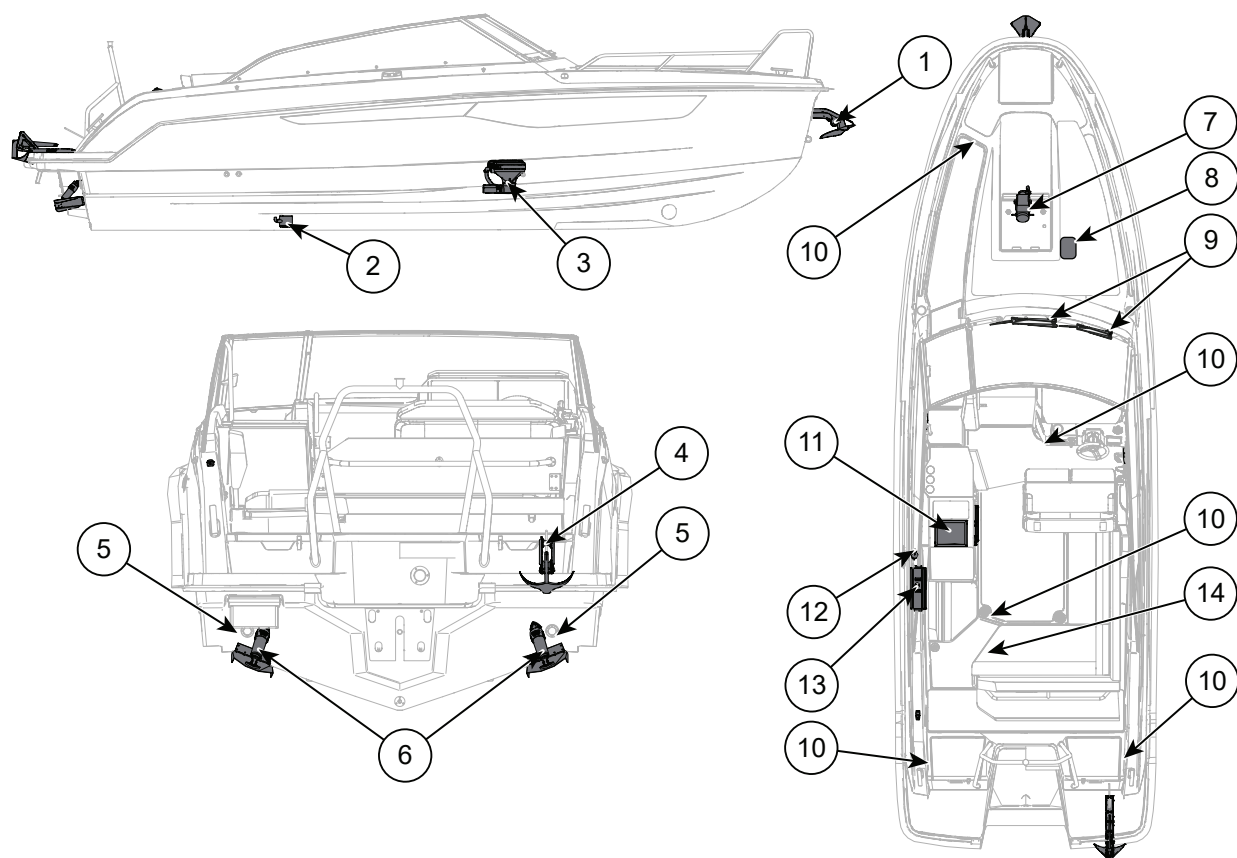
Figur 8.2 Yamarin 80 DC elektrisk utrustning
