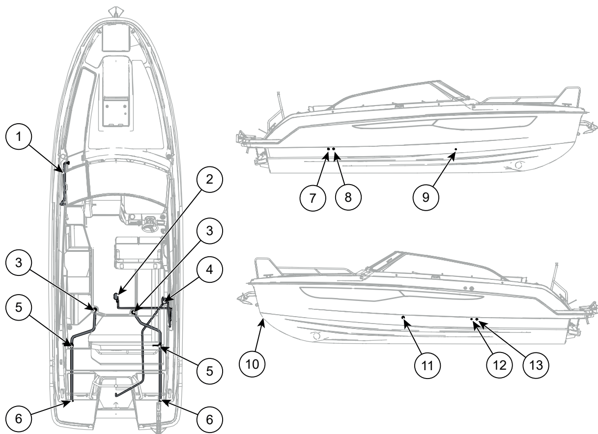
Figur 9.1 Yamarin 80 DC länspumpar och dränering
