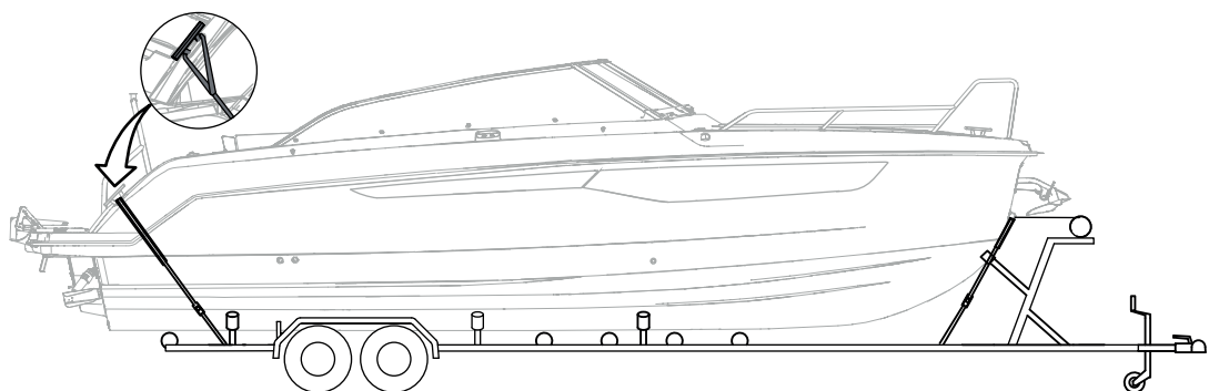
Figur 13.1 Yamarin 80 DC släpvagnstransport
