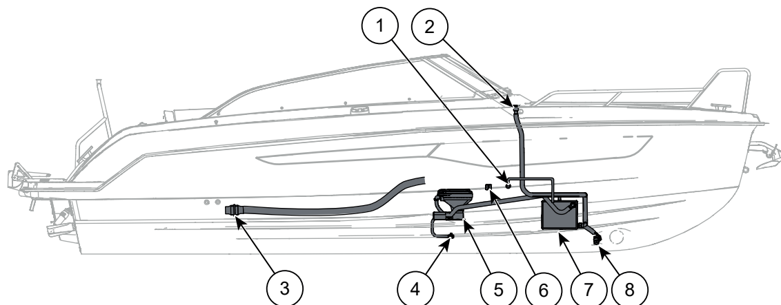
Figur 11.1 Yamarin 80 DC avloppssystem
