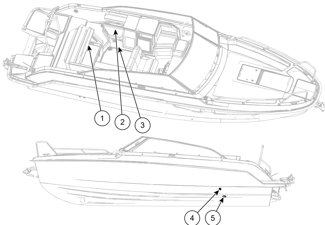
Figur 11.3 Yamarin 80 DC luftkonditioneringssystem
