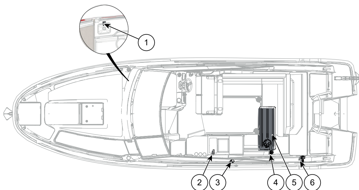
Figur 10.1 Yamarin 80 DC färskvattensystem
