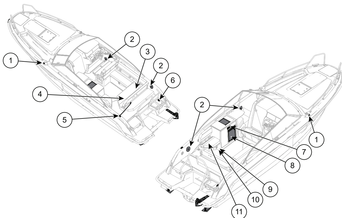
Figur 8.3 Yamarin 80 DC elektrisk utrustning
