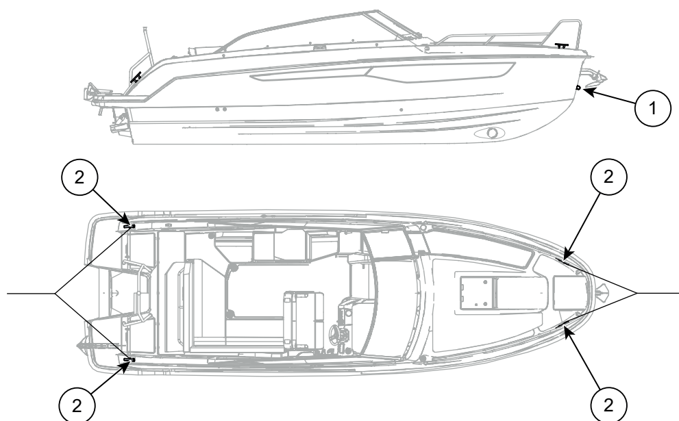
Figur 5.11 Yamarin 80 DC förtöjnings- och bogseringspunkter
