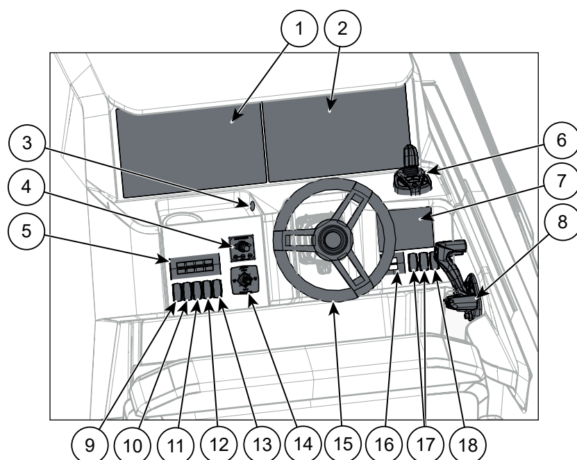
Figur 5.1 Yamarin 80 DC förarplatsens kontroller
