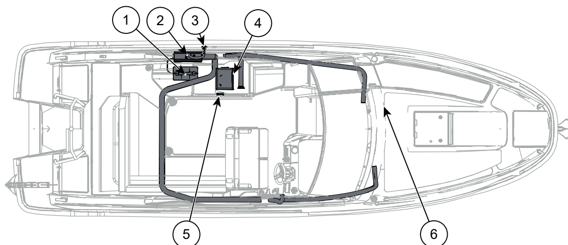
Figur 6.2 Yamarin 80 DC bränsle driven utrustning
