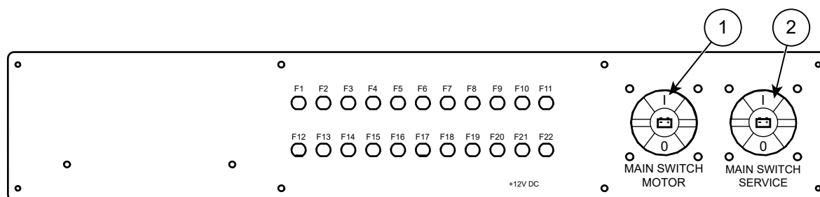
Figur 8.1 Yamarin 80 DC huvudströmbrytare och säkringspanel
