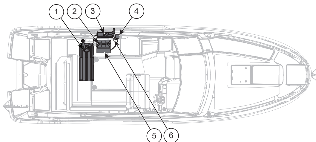
Figur 6.3 Yamarin 80 DC varmvattenberedare
